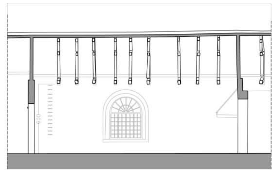
LONG SECTION B-B'
